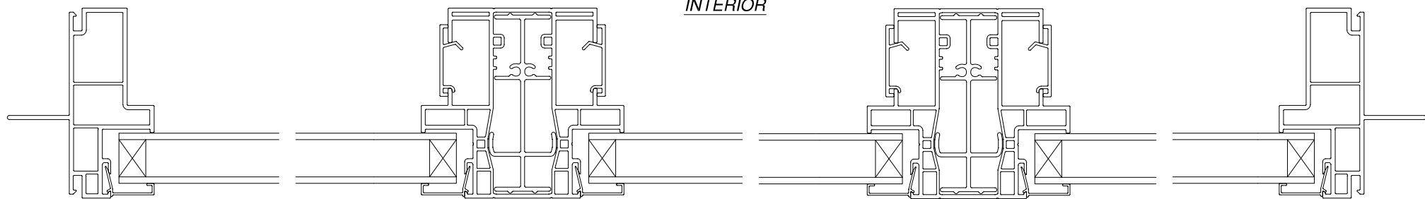
HORIZONTAL CROSS SECTION FIN FRAME
